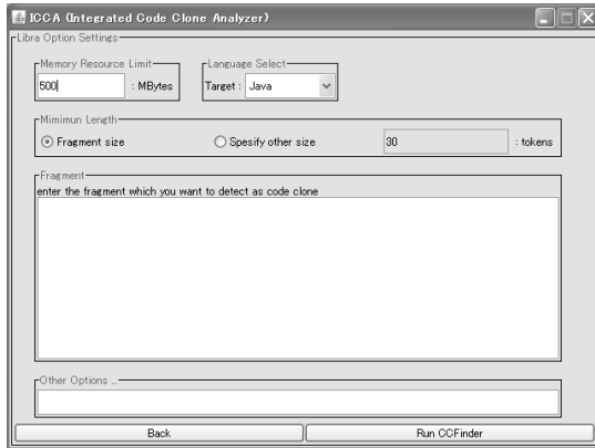
図 2 Libra のユーザインタフェース (検索条件指定画面) Fig. 2 A screen shot of Libra user interface. (search key specification screen)
