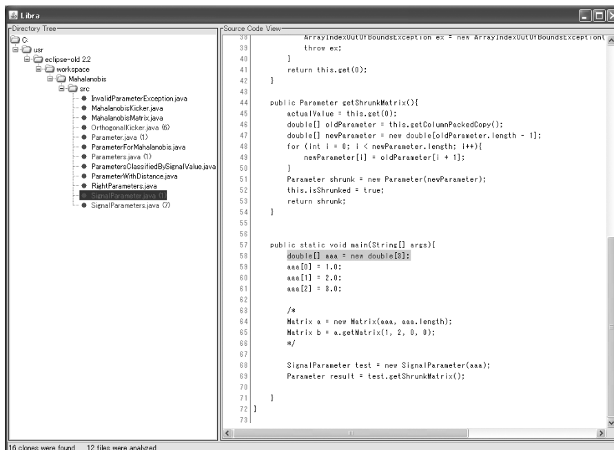
図 3 Libra のユーザインタフェース (検索結果表示画面) Fig. 3 A screen shot of Libra user interface. (search result screen)
