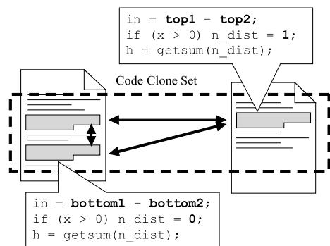
図 1 コードクローンとクローンセット
