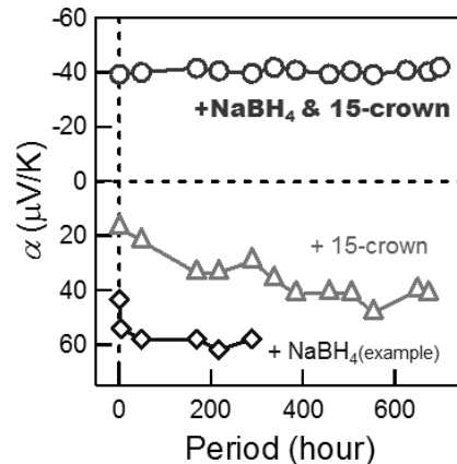
図3. クラウン錯体により配位したCNTのゼーベック係数、およびその大気安定性
