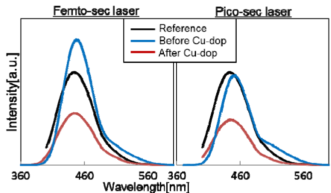
図 4 超短パルスレーザーを照射した ZnS 蛍光体の PL 発光スペクトル
