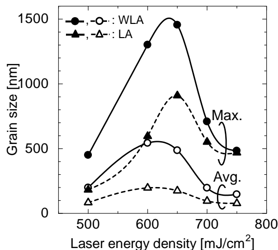
図 1 WLA/LA により形成した poly-Si 膜の最大粒径および平均粒径。
