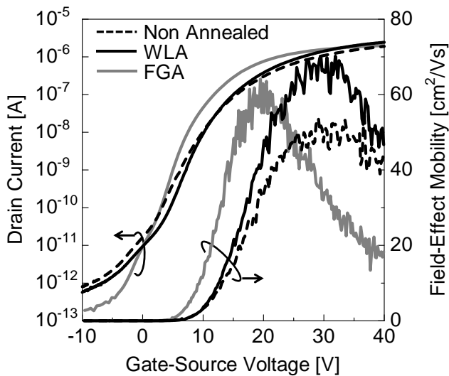
図 2 WLA/FGA 前後の poly-Si TFT の伝達特性。 V_{ds} = 0.1 \text{ V} , W/L = 5 \mu\text{m} / 10 \mu\text{m} .
