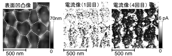
図 3 poly-Si 膜の表面凹凸像および電流像。
