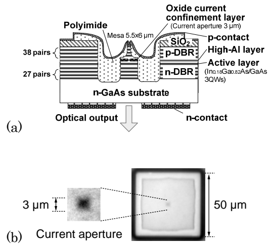
図 4. 酸化狭窄偏光双安定 VCSEL の構造 (a) と酸化狭窄構造の透過像 (b)
